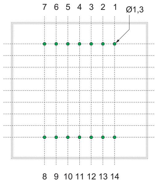
Ansicht auf Montageseite Raster = 5 mm Stiftquerschnitt = 0,8 x 0,6 mm Stiftlänge = 2,5 mm
