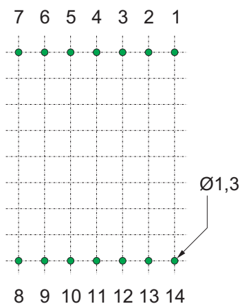
Ansicht auf Montageseite Raster = 5 mm Stiftquerschnitt = 0,8 x 0,6 mm Stiftlänge = 2,5 mm
