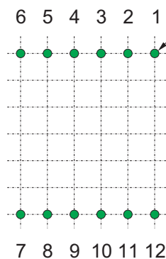
Ansicht auf Montageseite Raster = 5 mm Stiftquerschnitt = 0,6 x 0,8 mm Stiftlänge = 3,5 mm
