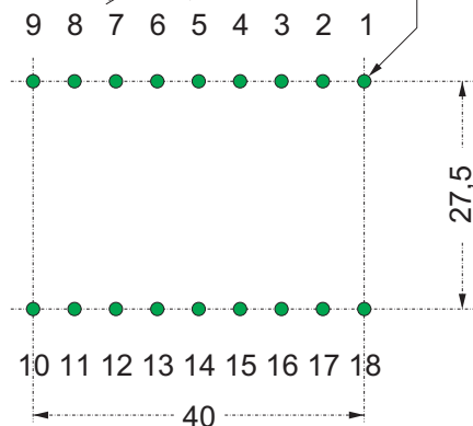
Ansicht auf Montageseite Stiftquerschnitt = 1,1 x 0,75 mm Stiftlänge = 3,5 mm
