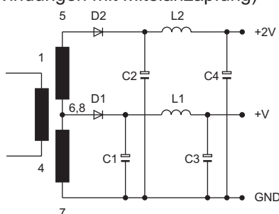
Schaltung C (Reihenschaltung der Windungen mit Mittelanzapfung)
