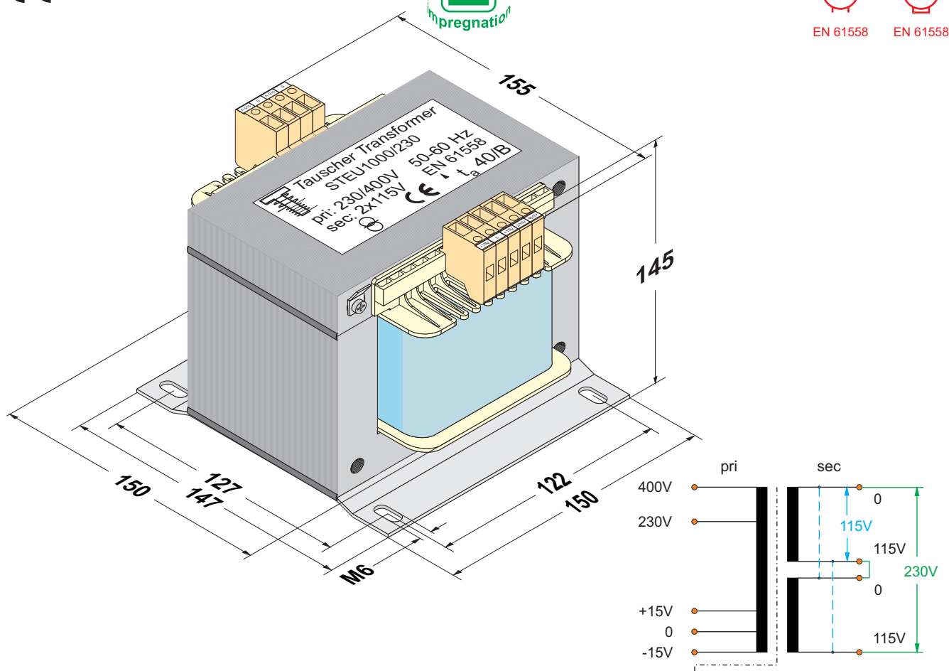
Reihenschaltung/series circuit: 230V 1x I sec Parallelschaltung/parallel circuit: 115V 2x I sec
